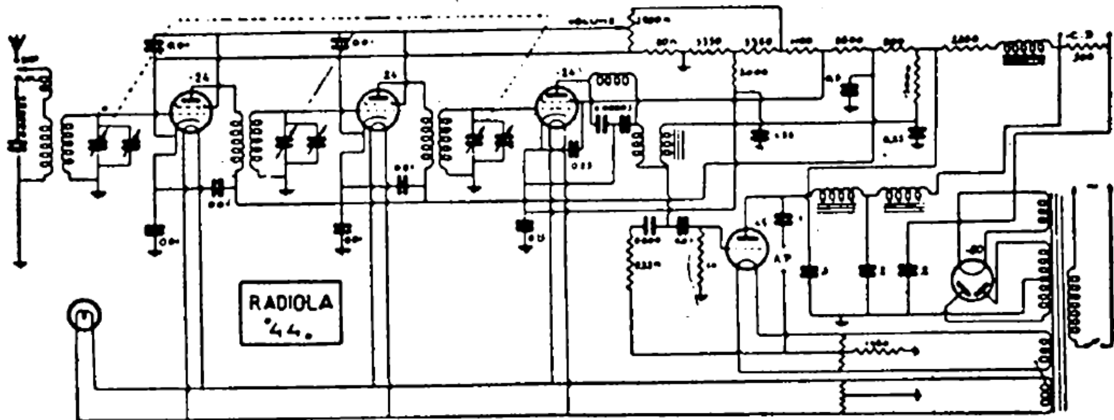
RCA (importaz. della C.O.E.). — Mod. Radiola 44. — Circuito ad amplificazione diretta. — Valvole e valori indicati nello schema. — Funzionava con diffusore magnetico e dinamico. — Controllo volume = 2900 ohm. — Produz. 1929-1930.
